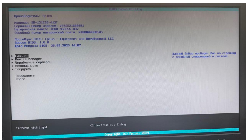
Рис. 2.1.1 – Приветственная форма
