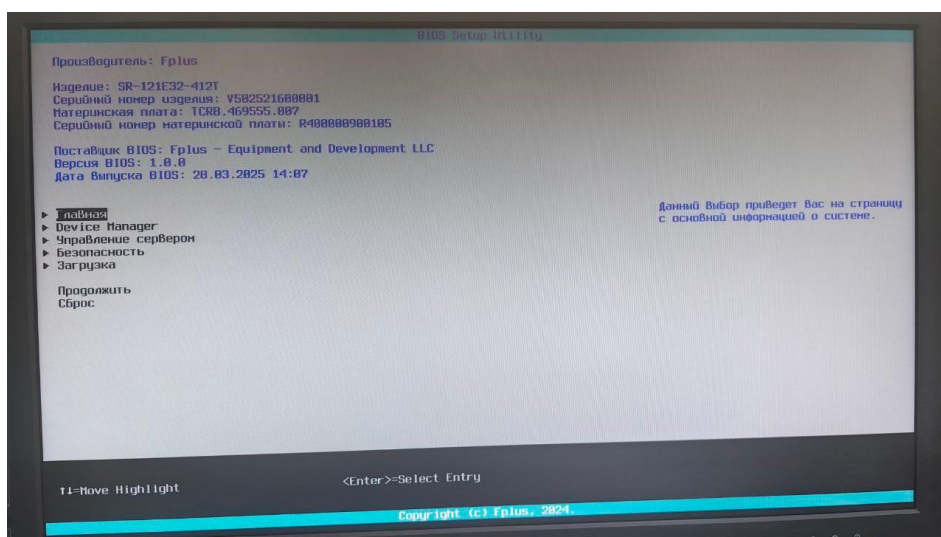
Рис. 2.1.1 – Приветственная форма
