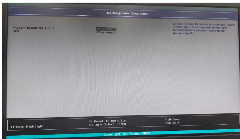
Рис. 2.5.1.1.1 - Конфигурация процессора
