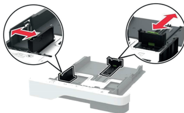
Рисунок 38 – Регулировка направляющих.
