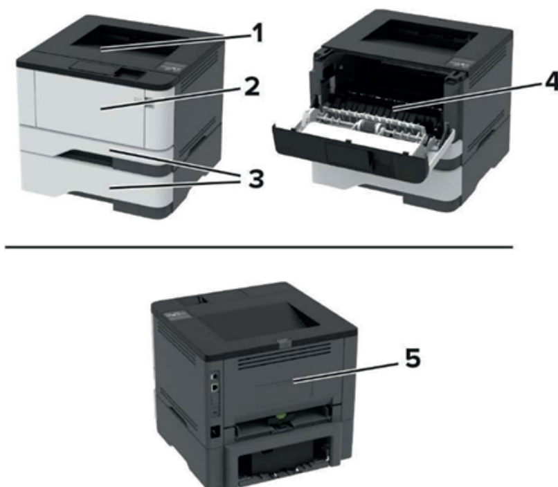
Рисунок 17 – Вероятные местоположения замятий.
