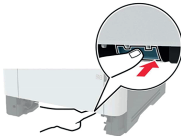
Рисунок 35 – Фиксатор устройства двусторонней печати.
