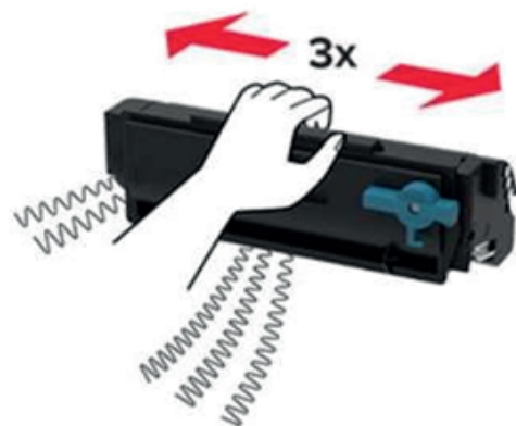
Рисунок 10 – Изображение встряхивания картриджа с тонером.
