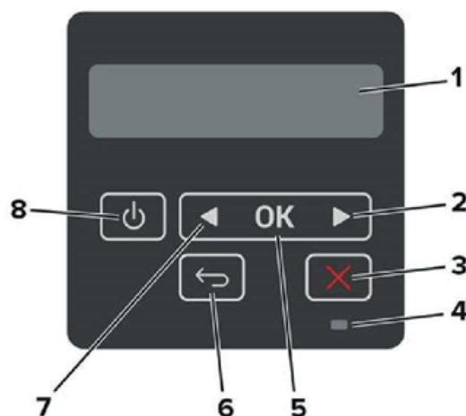
Рисунок 1 – Панель управления.
