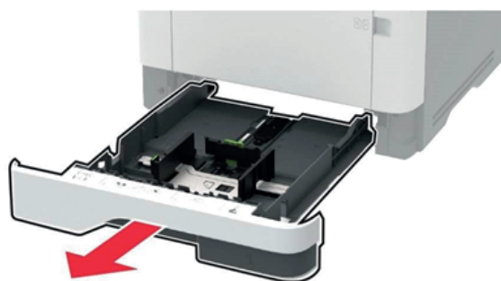
Рисунок 37 – Извлечение лотка.
